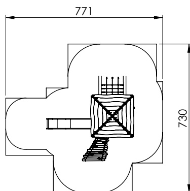
plattegrond
